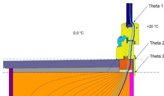
Fig. | Abb. 7: Posa filo interno | Einbau innenbündig
