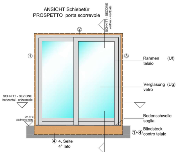
Fig. 2: Schema dell'alzante scorrevole Abb. 2 Schematische Darstellung HST
