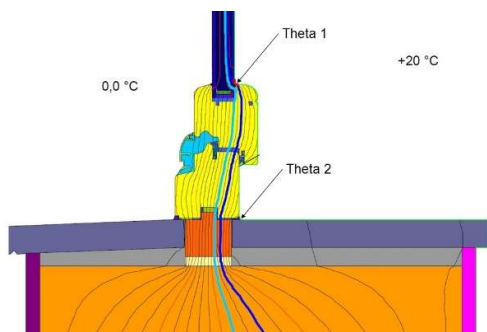
Fig. | Abb. 6: Posa centrale | Einbau mittig
